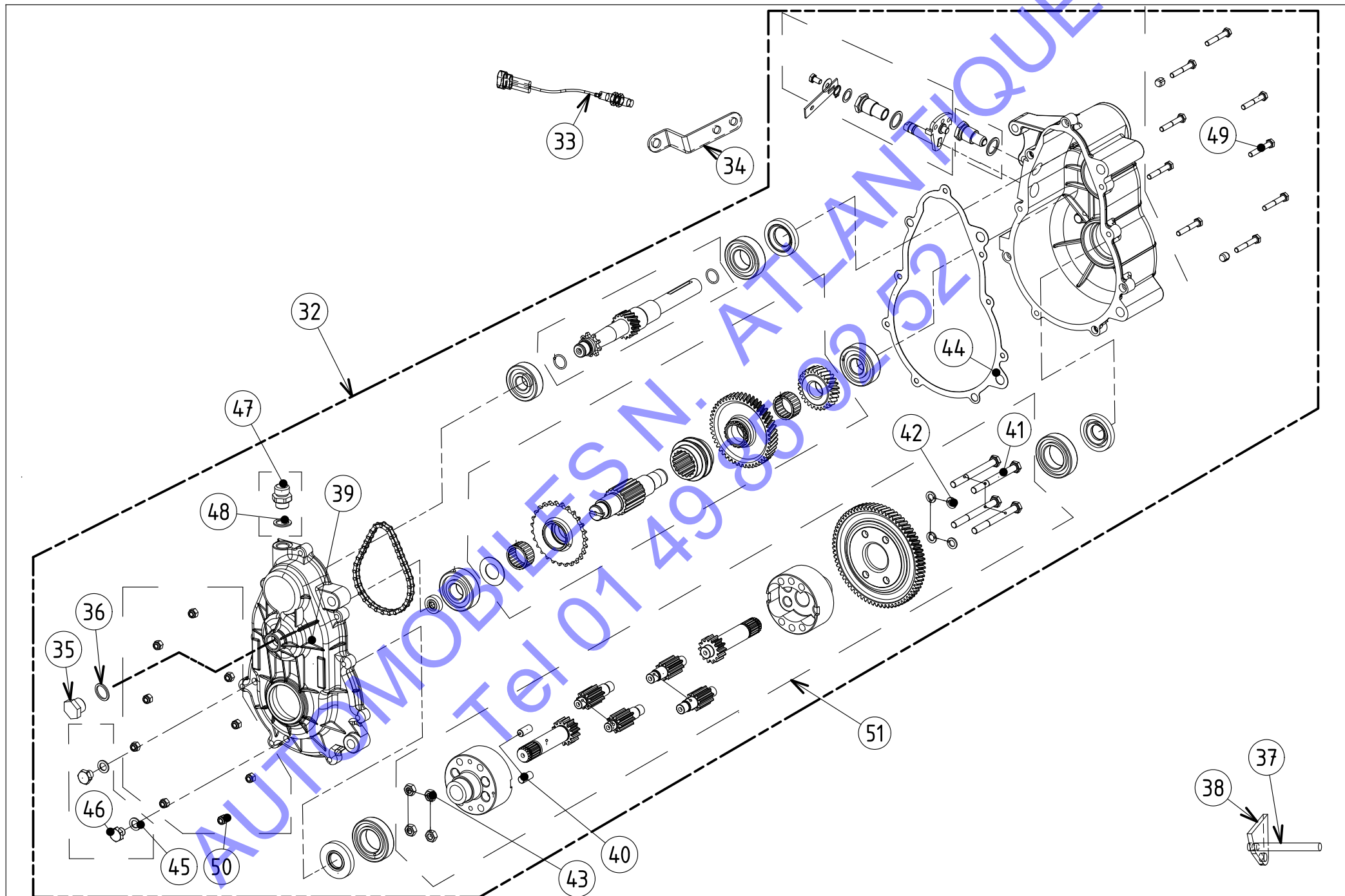
BOITE STILFRENI 1/8
